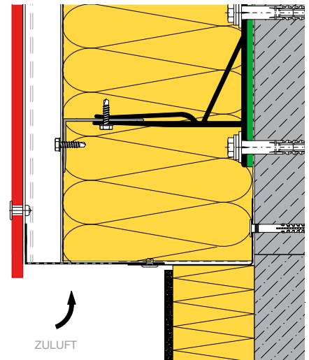
SOCKELANSCHLUSS A103
