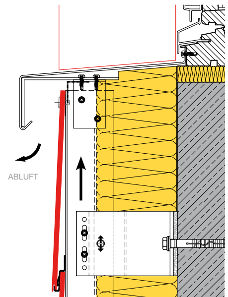
FENSTERBANKANSCHLUSS A102
