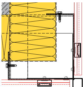
AUSSENECKE A105 MIT WÜRFELECKPROFIL
