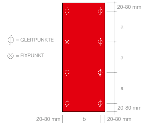
EINFELDPLATTE
