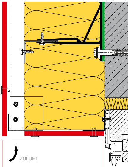
FENSTERSTURZ A101
