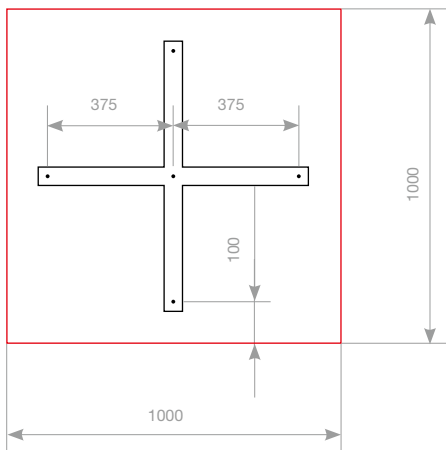
BEISPIEL TISCHPLATTEN-ÜBERSTÄNDE
