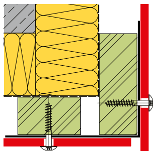
AUSSENECKE A105
