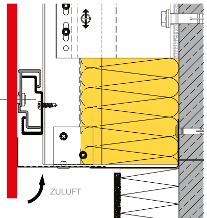
SOCKELANSCHLUSS A103
