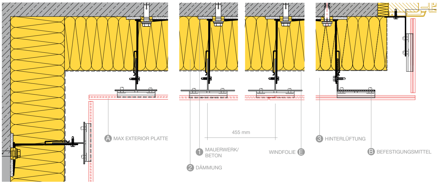
INNENECKE A106
