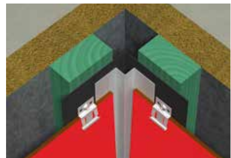
INNENECKE MIT INNENECKPROFIL
