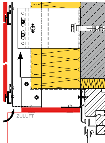
FENSTERSTURZ A101
