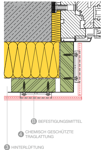
FENSTERLAIBUNG A104
