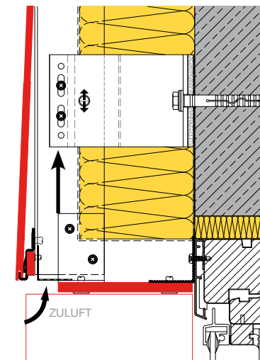
FENSTERSTURZ A101
