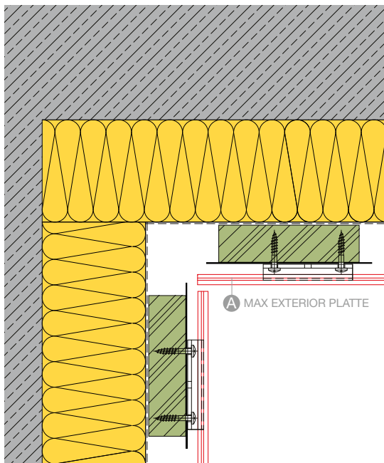
INNENECKE A106
