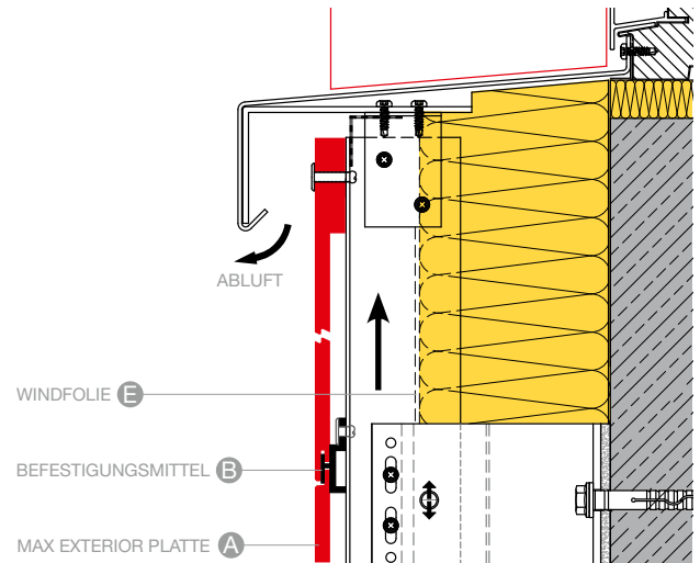
FENSTERBANKANSCHLUSS A102
