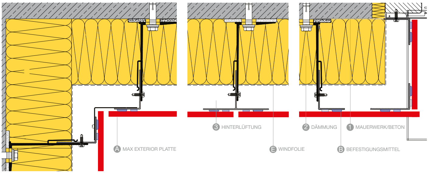
INNENECKE A106
