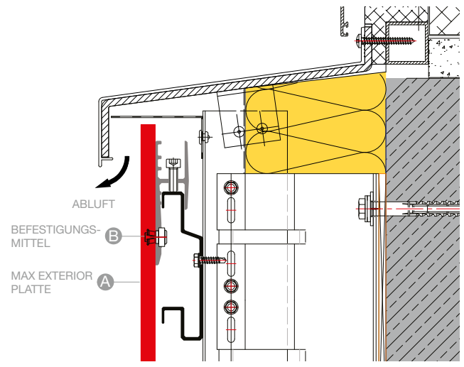
FENSTERBANKANSCHLUSS A102
