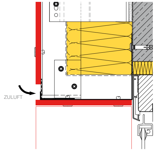
FENSTERSTURZ A101.2*
