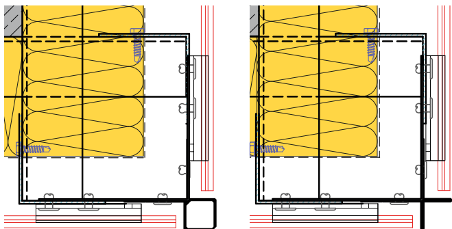
AUSSENECKE A105 MIT WÜRFLECKPROFIL
