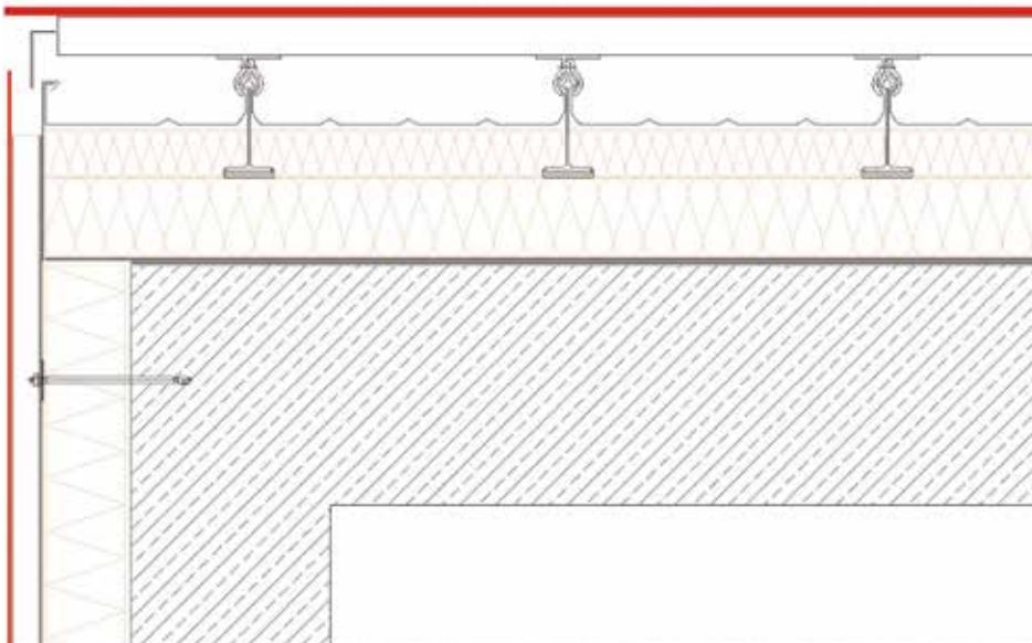
LOTSCHNITT ORTGANG
