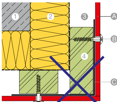
WAAGSCHNITT
