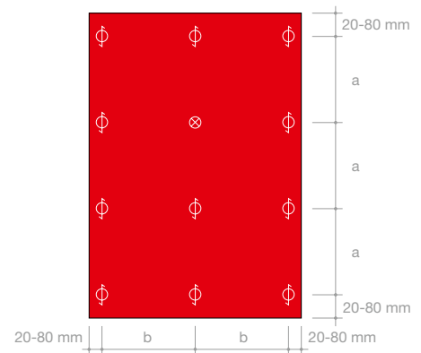
ZWEIFELDPLATTE
