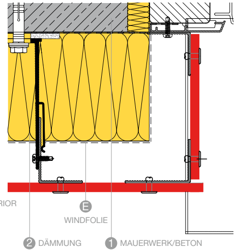
FENSTERLAIBUNG A104
