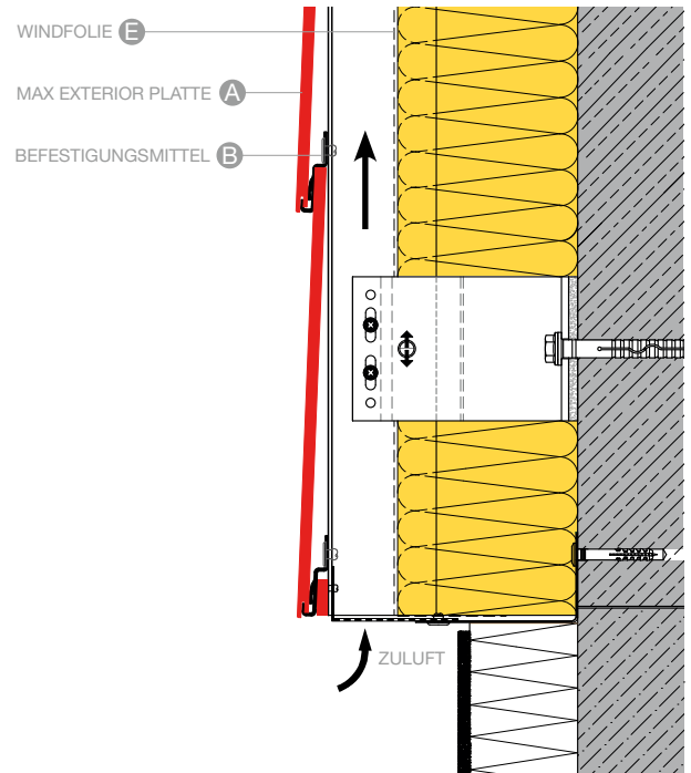
SOCKELANSCHLUSS A103
