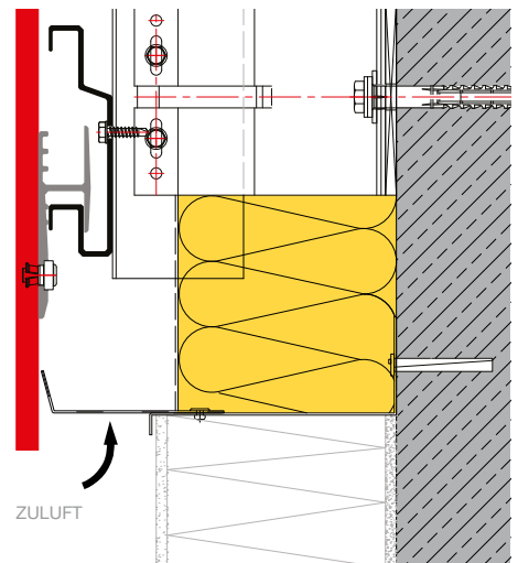
SOCKELANSCHLUSS A103
