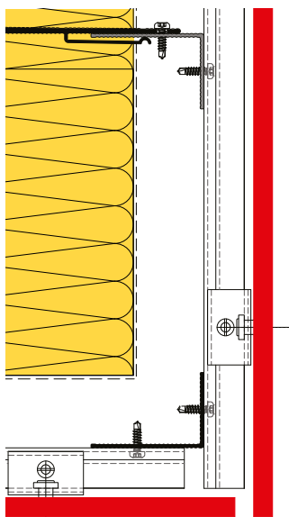
AUSSENECKE A105
