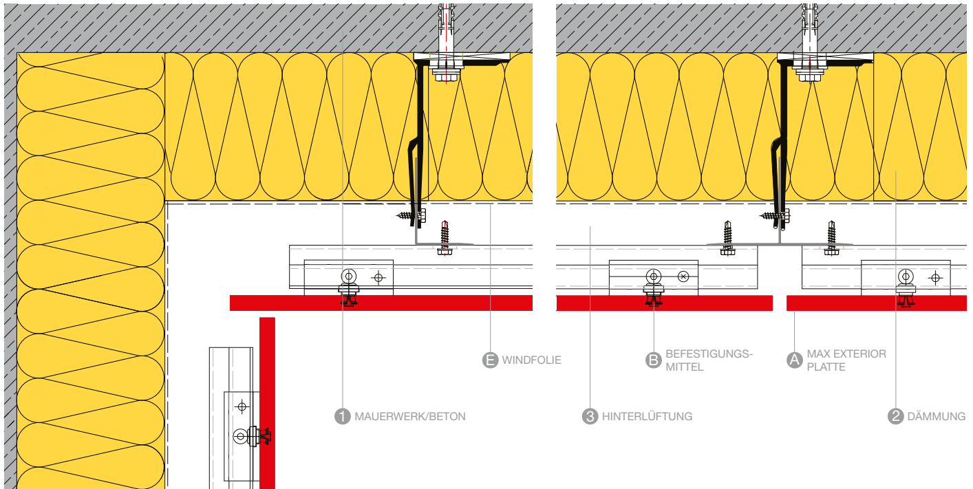
INNENECKE A106
