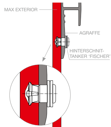
DETAIL HINTERSCHNITTANKER
