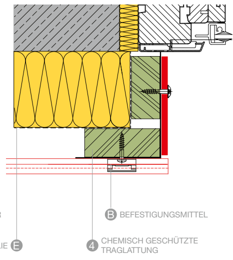
FENSTERLAIBUNG A104
