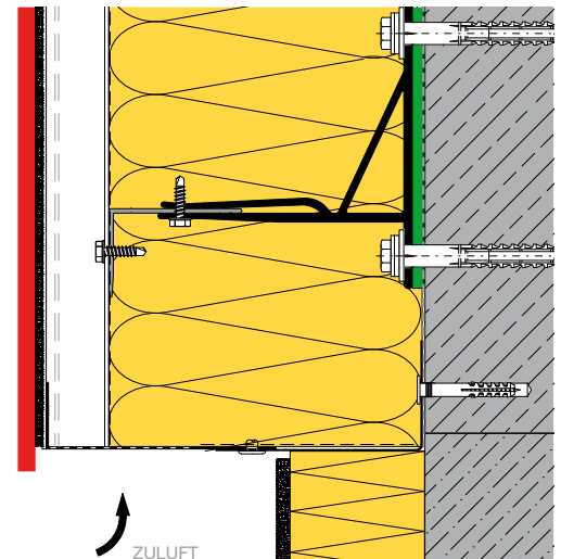
SOCKELANSCHLUSS A103
