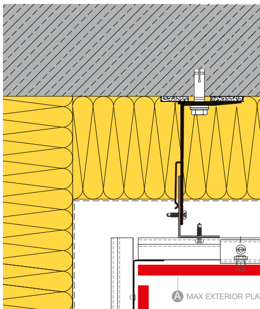
INNENECKE A106
