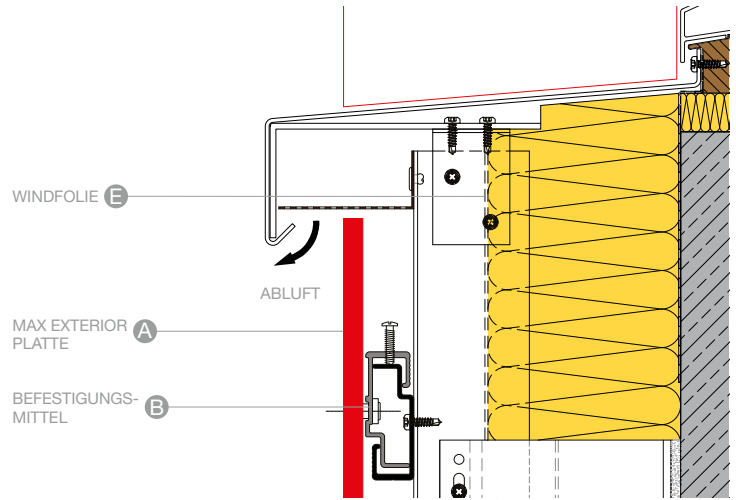
FENSTERBANKANSCHLUSS A102
