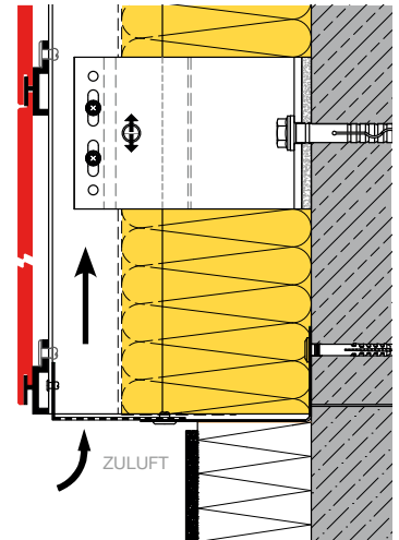
SOCKELANSCHLUSS A103
