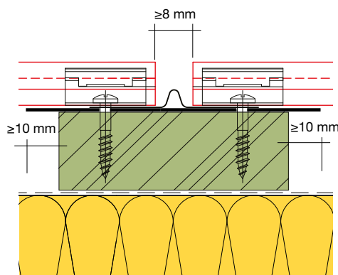
FUGENHINTERLEGUNGSPROFIL
