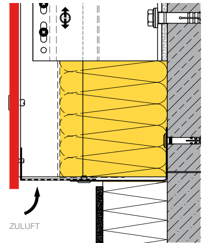
SOCKELANSCHLUSS A103
