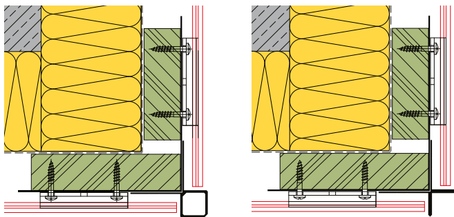
AUSSENECKE A105 MIT WÜRFELECKPROFIL
