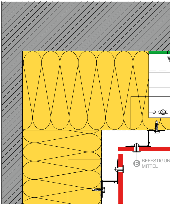
INNENECKE A106
