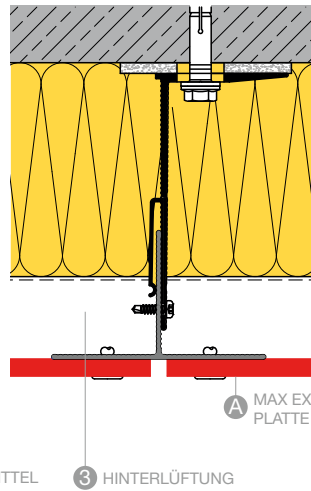
VERTIKALFUGE A107
