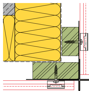
AUSSENECKE A105 MIT KREUZECKPROFIL
